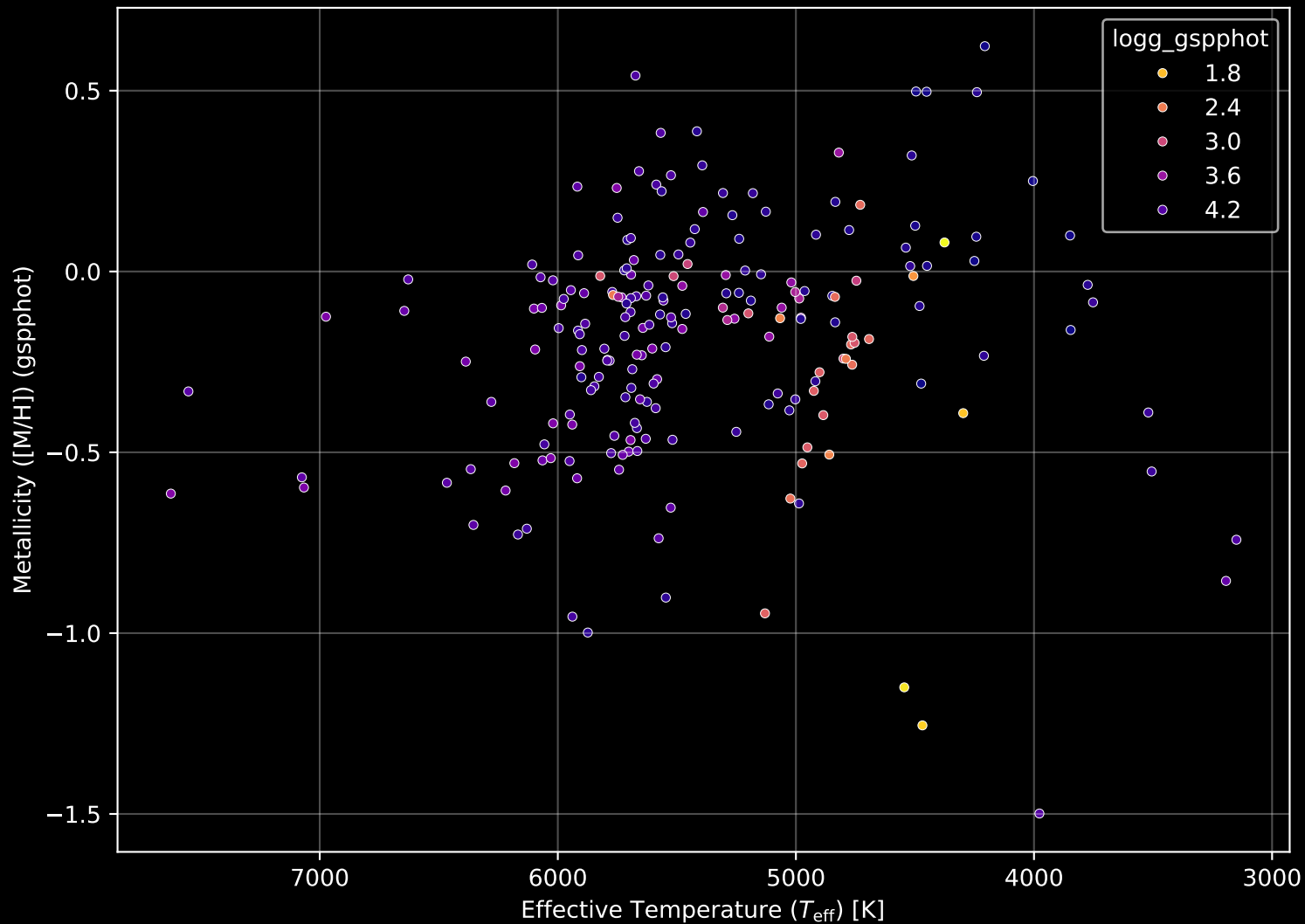
APOGEE DR17 Field: [270-40-O_TESS] Stellar Population Parameters (n= 208)
